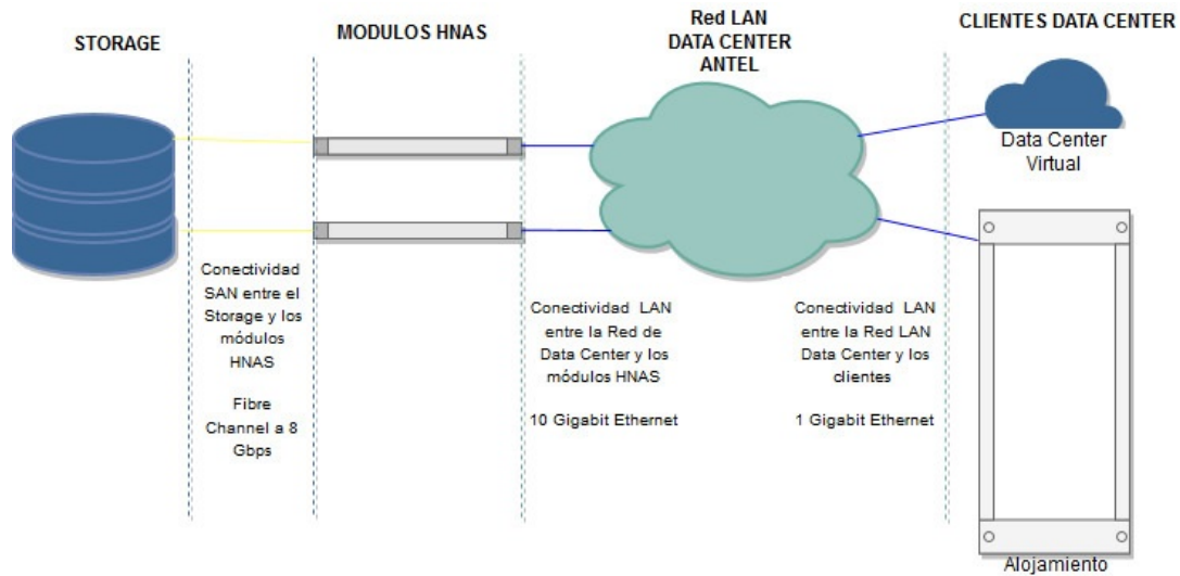
Imagen 1- Topología
